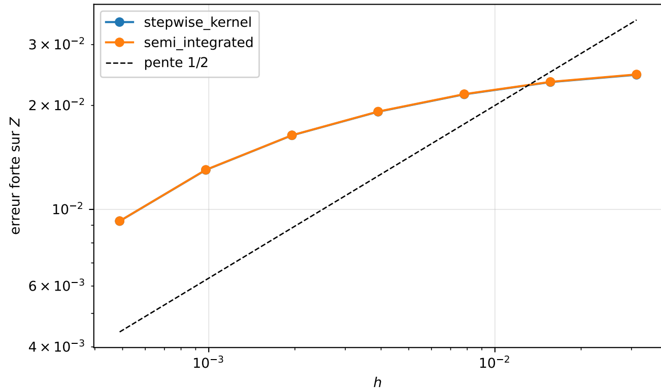
Comparaison des deux variantes du pseudo-Euler
