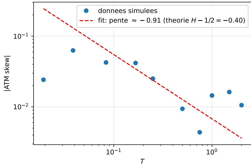
Echelle log-log : verification de la loi de puissance
